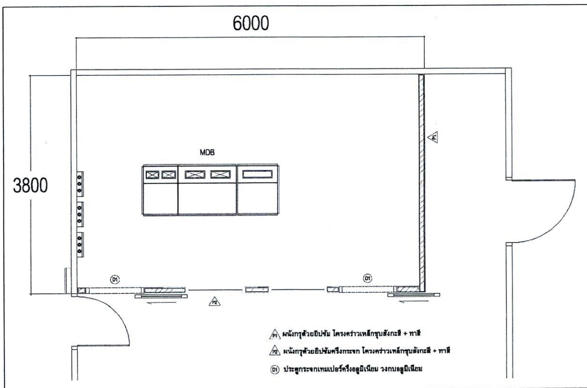
ภาพแสดงห้องเครื่องจ่ายกระแสไฟฟ้าสำรองต่อเนื่อง (UPS)
