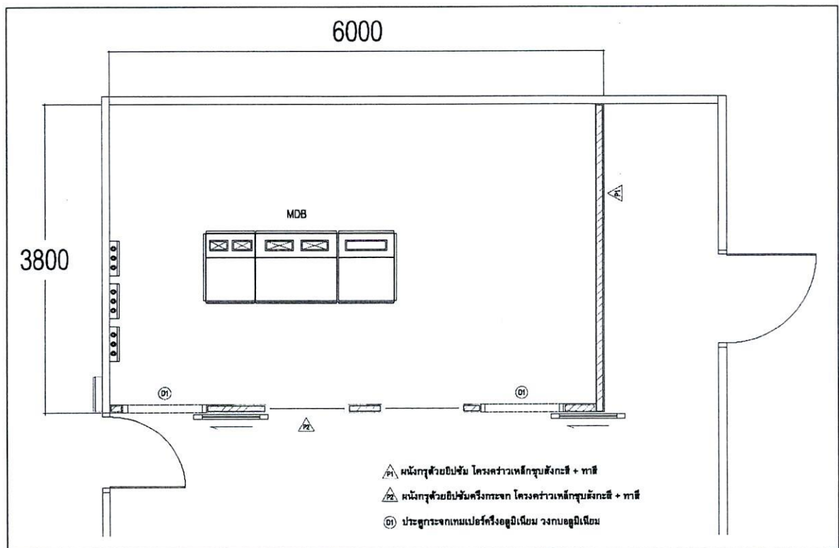
ภาพแสดงห้องเครื่องจ่ายกระแสไฟฟ้าสำรองต่อเนื่อง (UPS)
