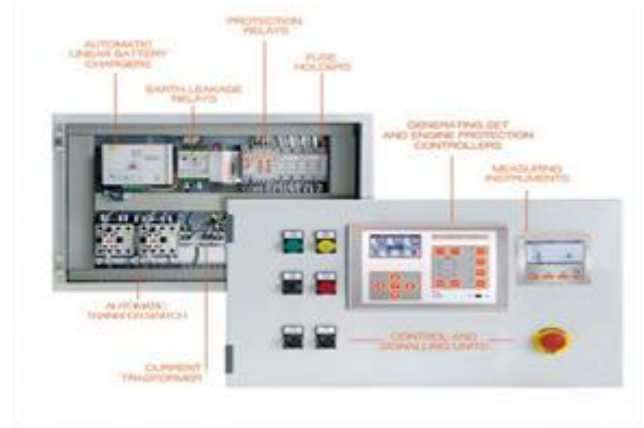
ภาพ ระบบไฟฟ้าสำรองเพื่อรองรับสถานการณ์ฉุกเฉินและจำเป็นในการกิจด้านเทคโนโลยีสารสนเทศ และการสื่อสาร
